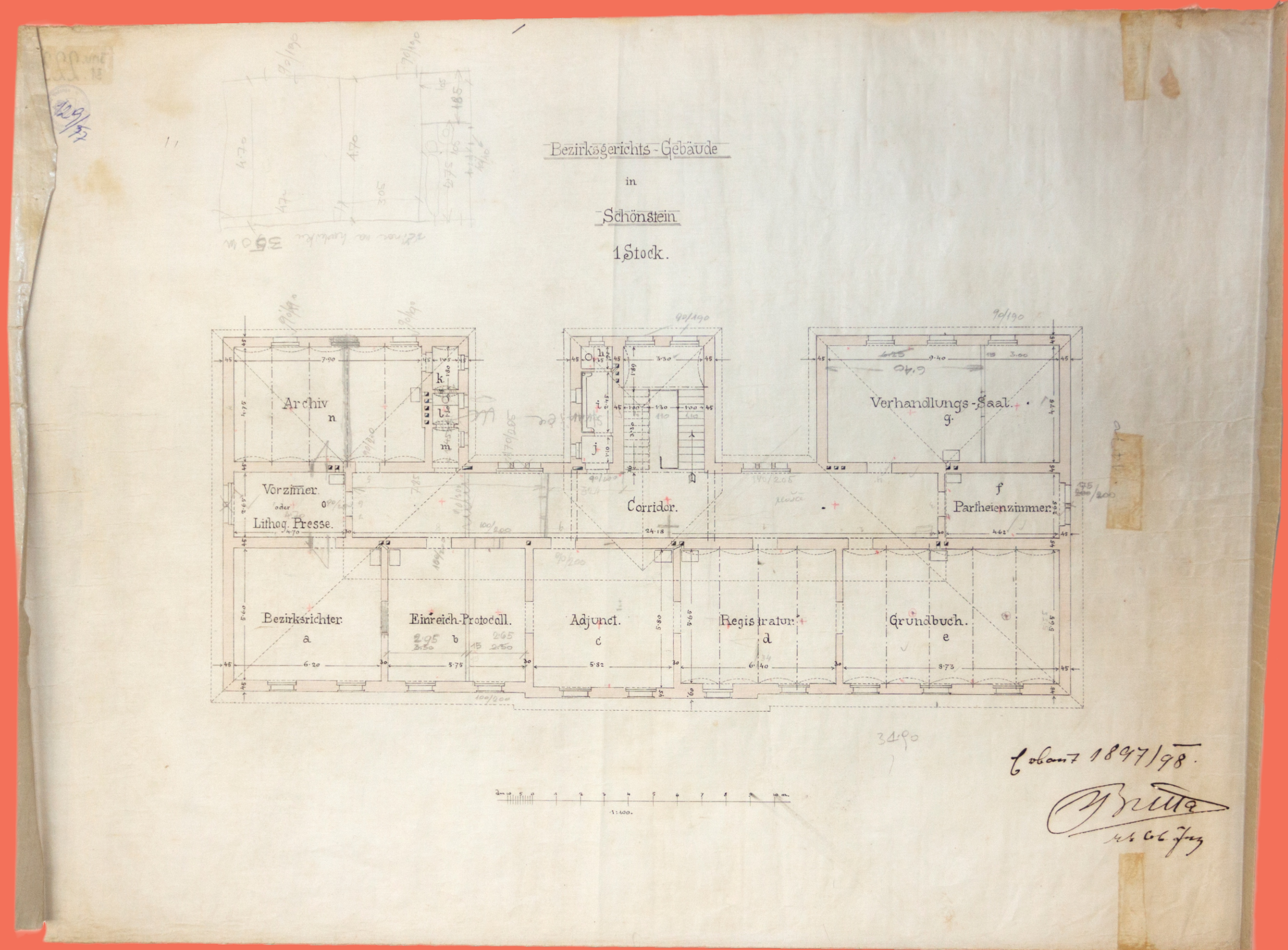
Tloris prvega nadstropja (1. Stock) sodiščne palače. V zgornjem nadstropju so se nahajale pisarne za sodnike, sodna dvorana, registratura, prostori za zemljiško knjigo in sodiščni arhiv. Digitaliziran načrt hrani avtor, original Muzej Velenje.
