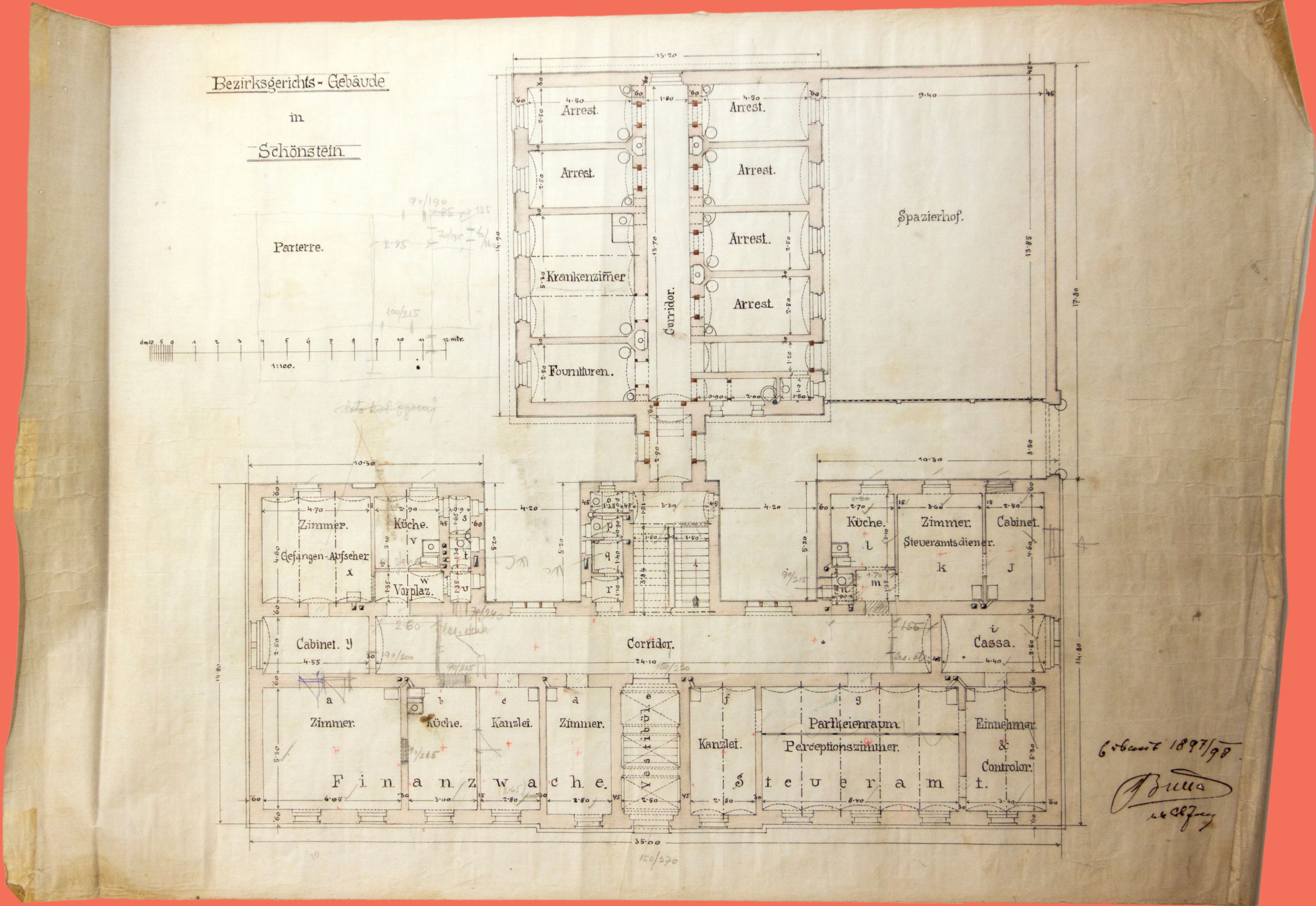
Tloris pritličja (Parterre) sodiščne palače Okrajnega sodišča v Šoštanju. Stavba, zgrajena v letu 1897/98 predstavlja tipično sodno palačo poznega 19. stoletja. V pritličju sta se poleg pisarn nahajali še stanovanji davčno-finančnega policista in zaporniškega predstojnika. Iz osrednjega stopnišča je vodil hodnik v prizidek s šestimi celicami, bolnišnično sobo in shrambo ter zaprtim dvoriščem za pripornike. Digitaliziran načrt hrani avtor, original Muzej Velenje.
